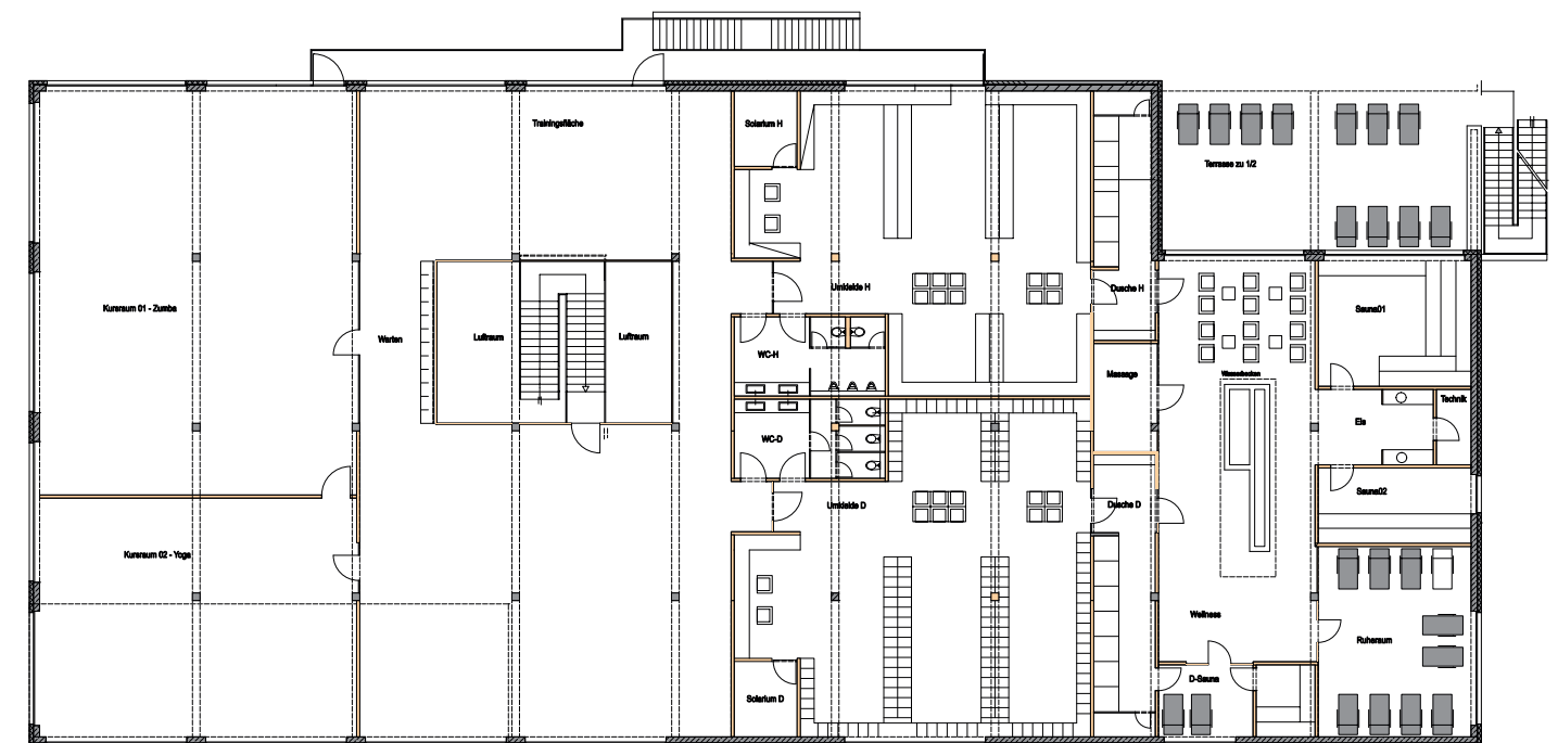
Obergeschoss
